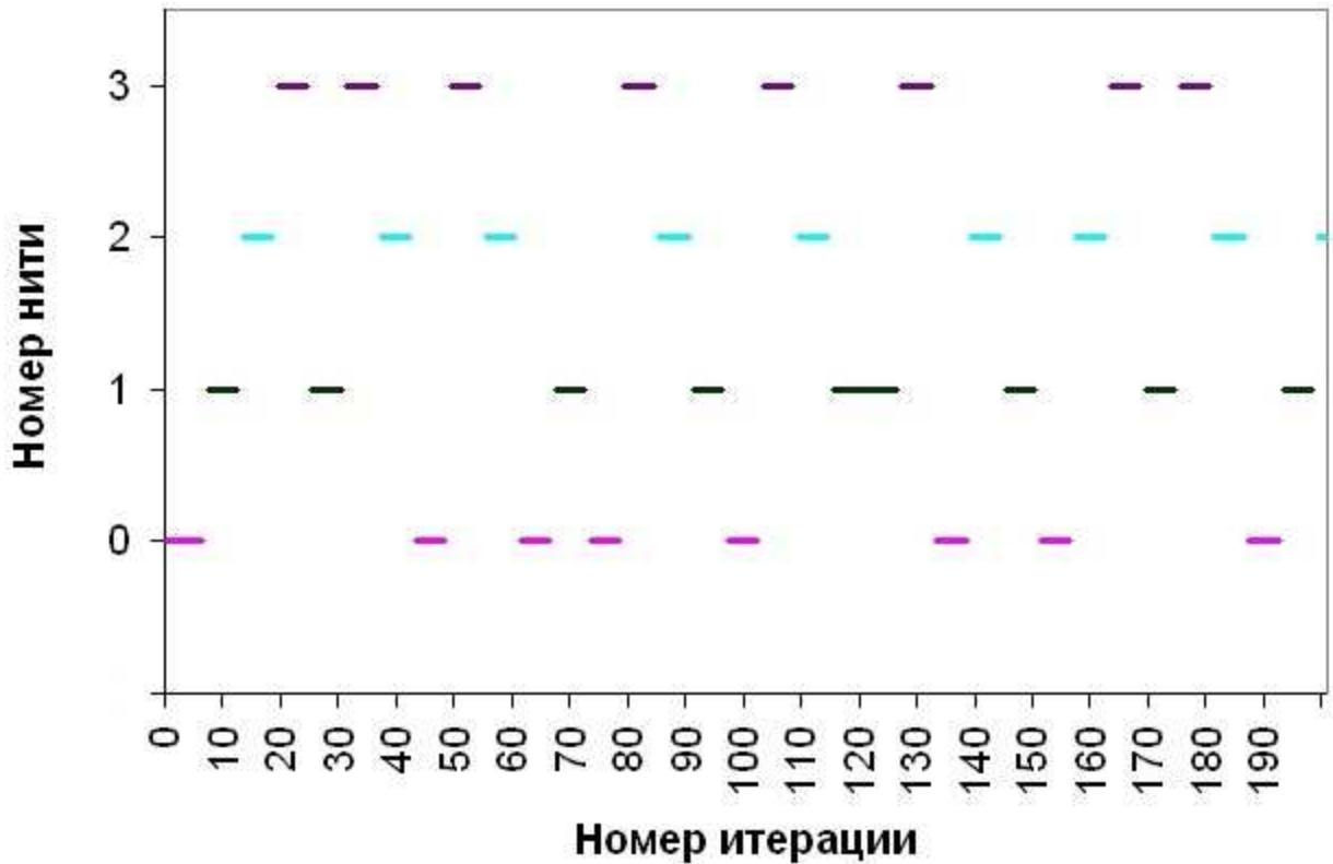
Рис.1б. Распределение итераций по нитям для ( dynamic , б)
