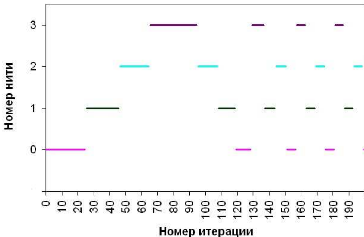
Рис.1с. Распределение итераций по нитям для (guided, 6)
