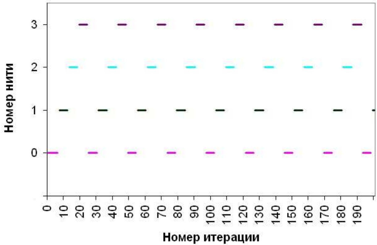
Рис.1а. Распределение итераций по нитям для ( static , б)
